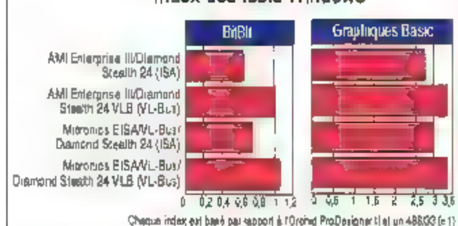
Figure 2 - Test vidéo des deux cartes mères en utilisation ISA et VL-Bus. Le test BIBI totalement montre un accroissement des performances très important lorsqu'on l'exécute sur une carte vidéo VL-Bus.
